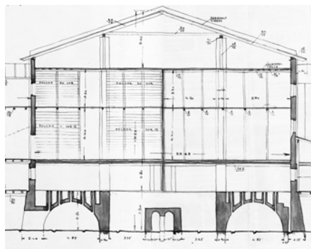
Körkemence és műszárító épületének metszete
